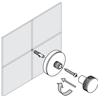
Установка вешалки «Каньон»
