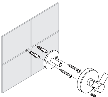
Установка вешалки «Виктория»
